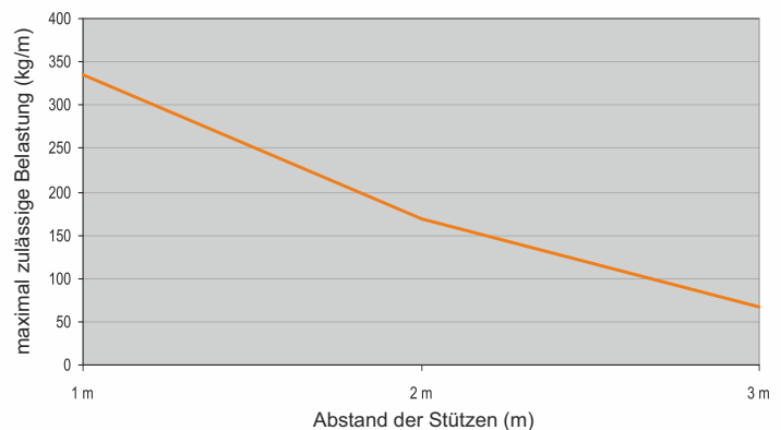
Der Graf zeigt die maximal zulässige gleichmäßige Belastung der Leiter im Verhältnis zu den Stützenabständen.
